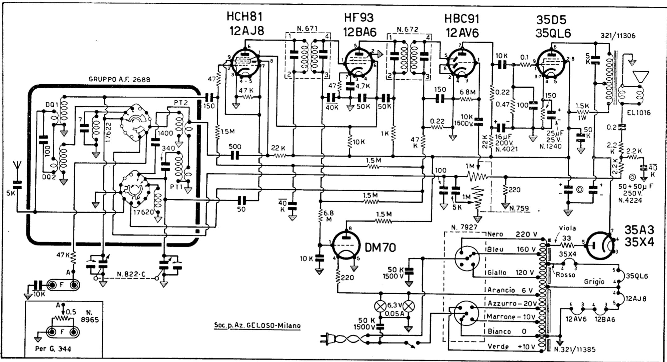
Schema elettrico dei ricevitori G 332 e G 344
